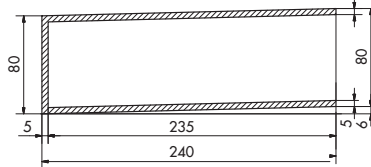
SEZIONE LATERALE
