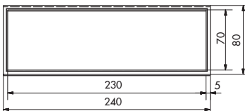
PIANTA
