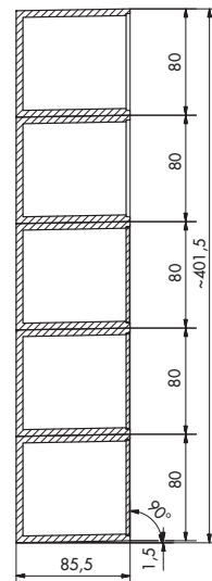
SCHEMA DI MONTAGGIO (composizione massima 5 posti)
