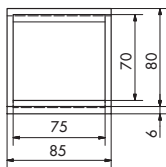
SEZIONE FRONTALE
