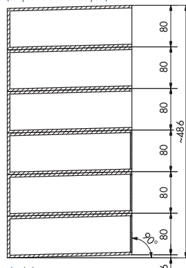
SCHEMA DI MONTAGGIO (composizione massima 6 posti)
