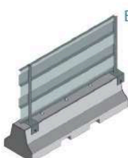
MONTAGGIO DI PIANTANE SINGOLE
